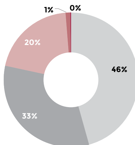
Inundações
