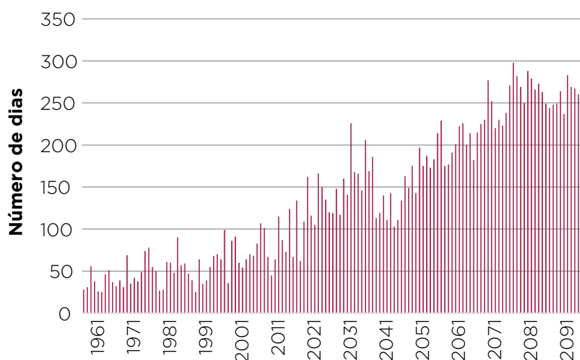
Figura 10 – Número projetado de dias com um Índice de Calor acima de 40°C, como modelado pelo HADGEM2-ES sob o cenário RCP 8.5
