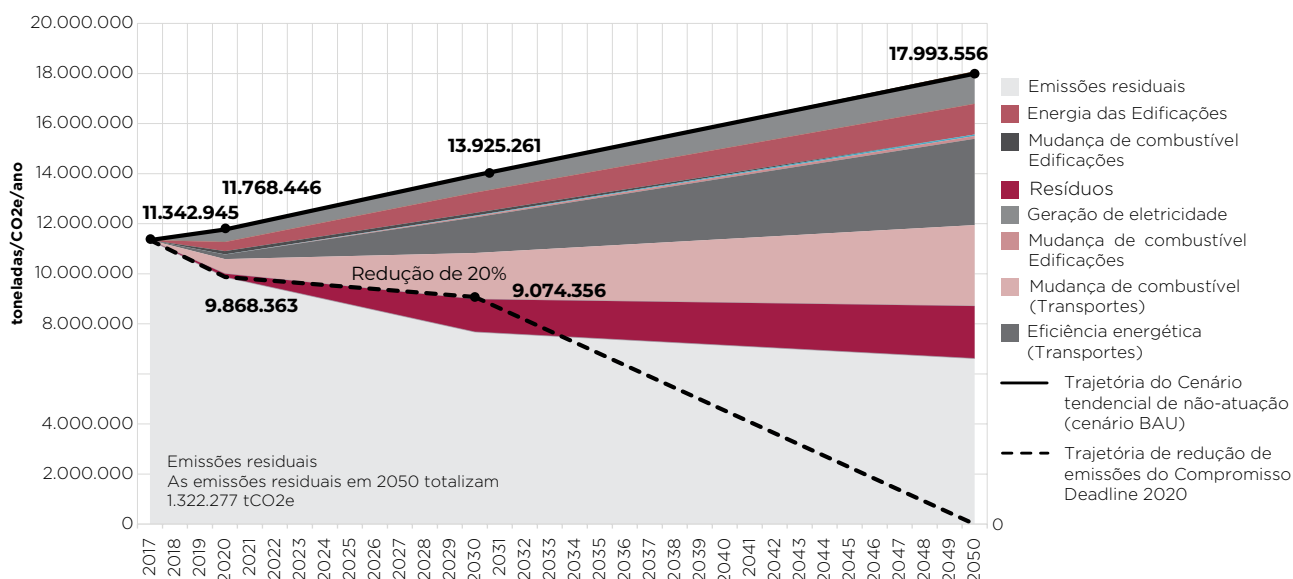
Figura 8 – Gráfico da trajetória de redução de emissões por setor no Cenário Ambicioso. O valor de 20% indica a meta de redução de emissões assumida pela cidade neste Plano
