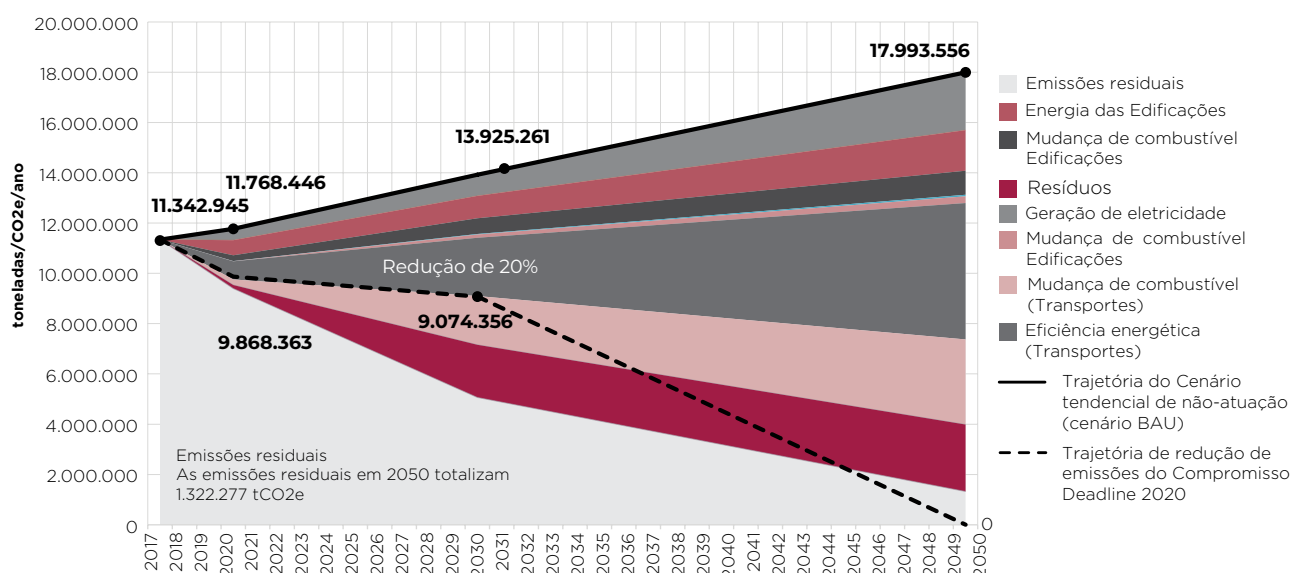
Figura 9 - Gráfico da trajetória de redução de emissões por setor no Cenário de Máxima Ambição
