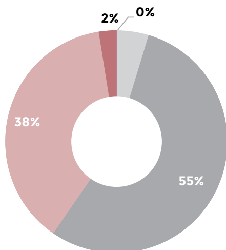
Onda de Calor
