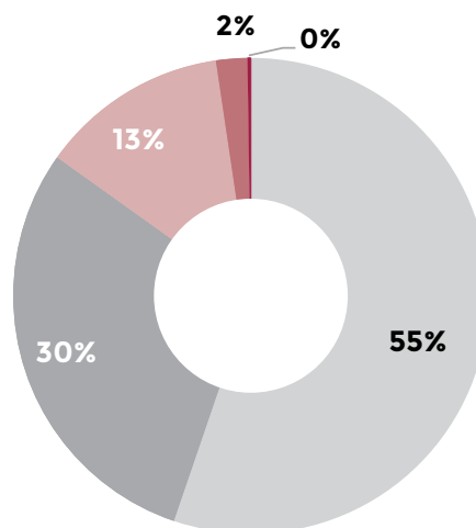
Deslizamentos
