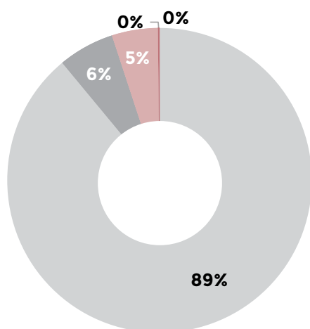
Elevação do nível médio do mar
