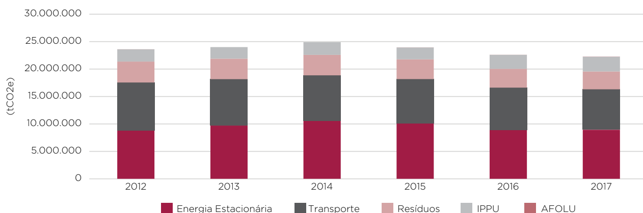
Figura 6 – Emissões de Gases de Efeito Estufa (tCO 2 e) da Cidade do Rio de Janeiro por ano e por setores – 2012 a 2017
