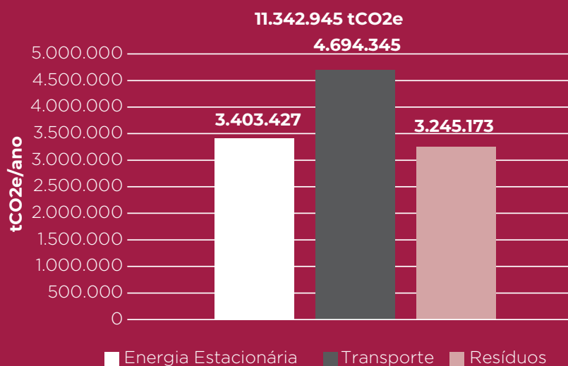
Figura 7 – Total de emissões dos Setores BASIC para o ano-base de 2017, para a ferramenta Pathways
